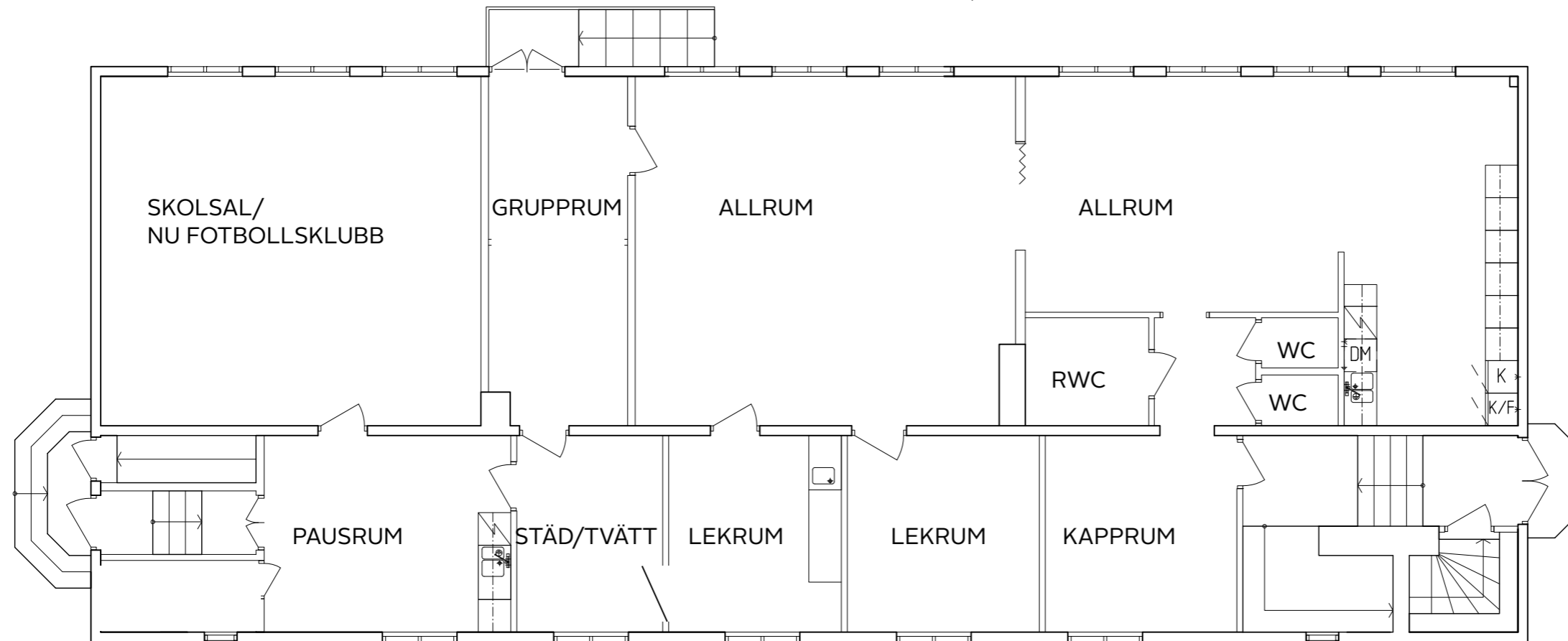
ENTRÉPLAN
